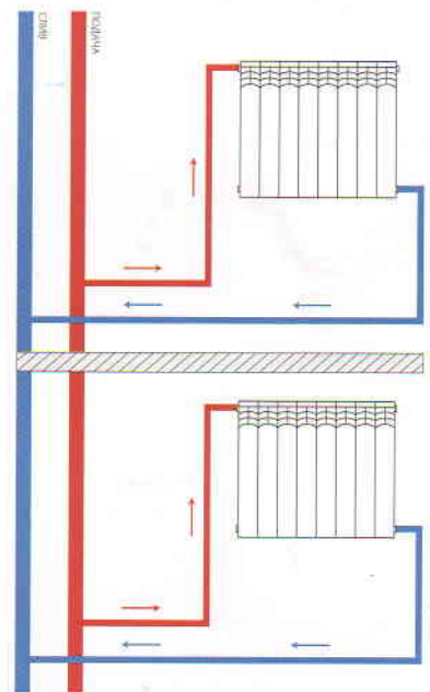
Двухтрубное подключение в вертикальном трубопроводе
