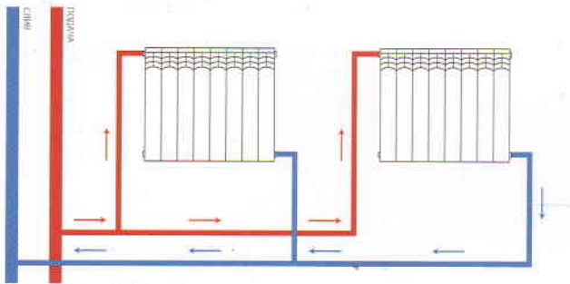
Двухтрубное подключение в горизонтальном трубопроводе
