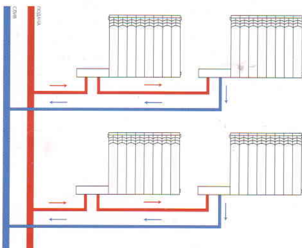
Однотрубное подключение
